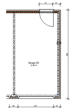
3 rez-de-chaussee, garage G5 1 : 50
