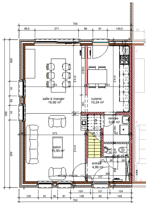
1 rez-de-chaussee 1 : 50
