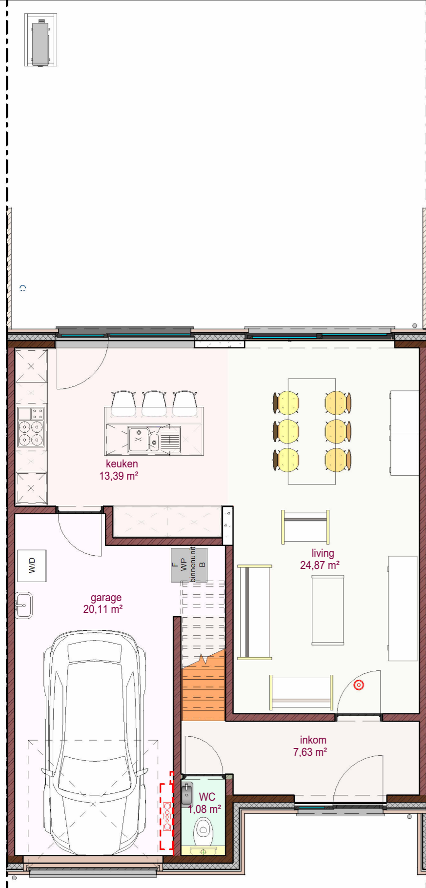
1 Gelijkvloers 178 LL 1 : 70
