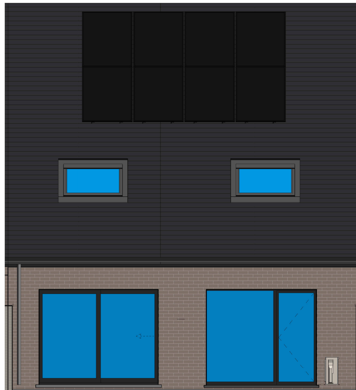
LL Achtergevel lot 178
