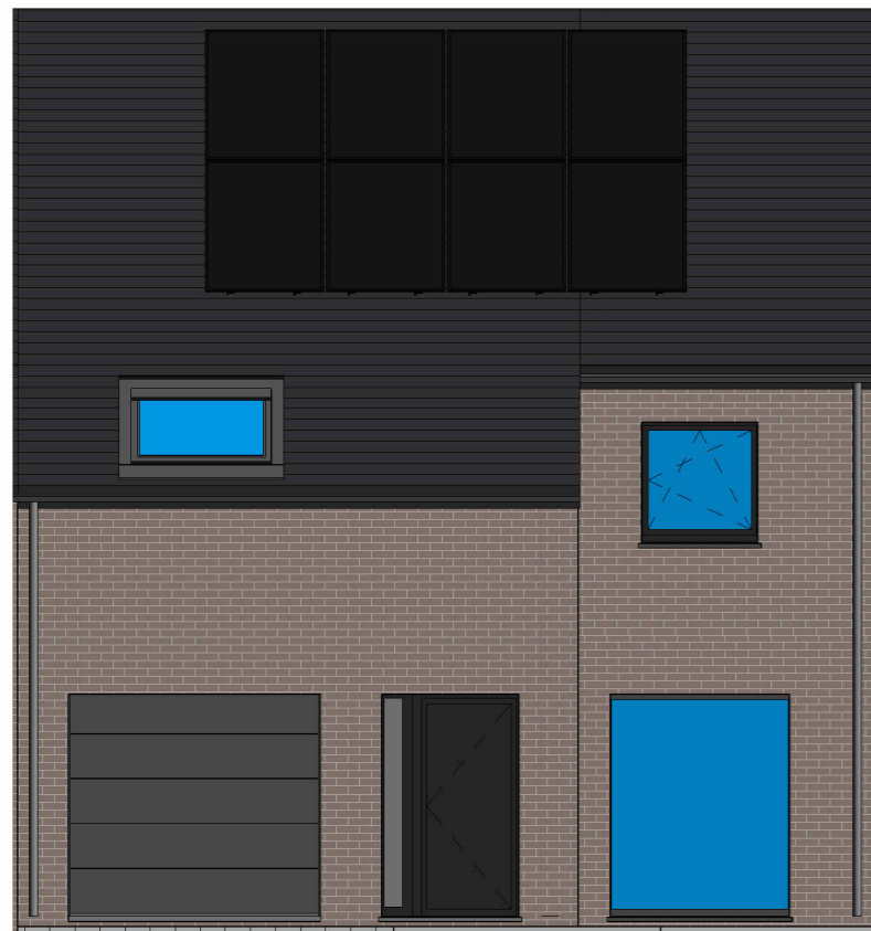
LL Voorgevel lot 180
