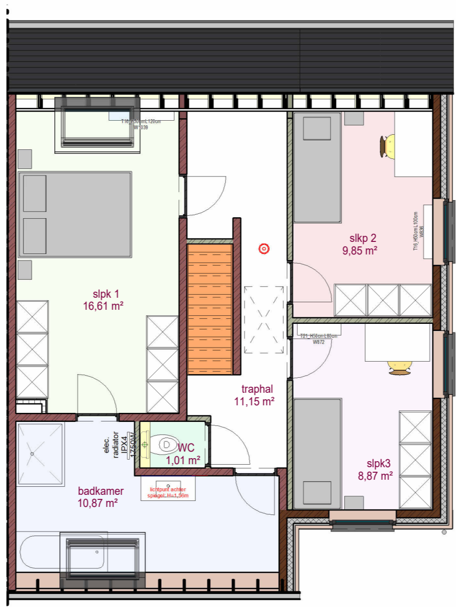
2 Verdieping 180 LL 1 : 70
