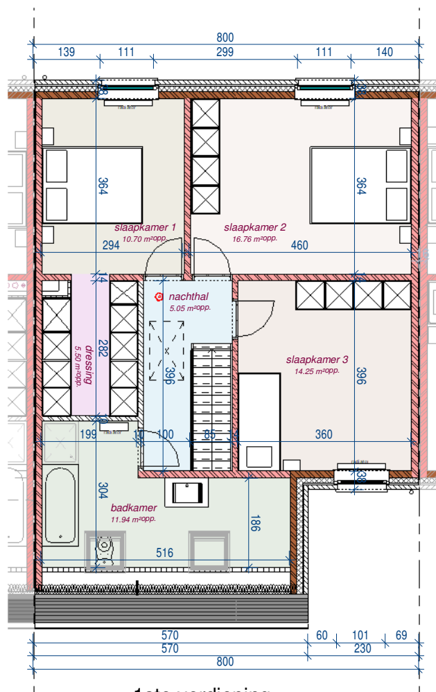
1ste verdieping
