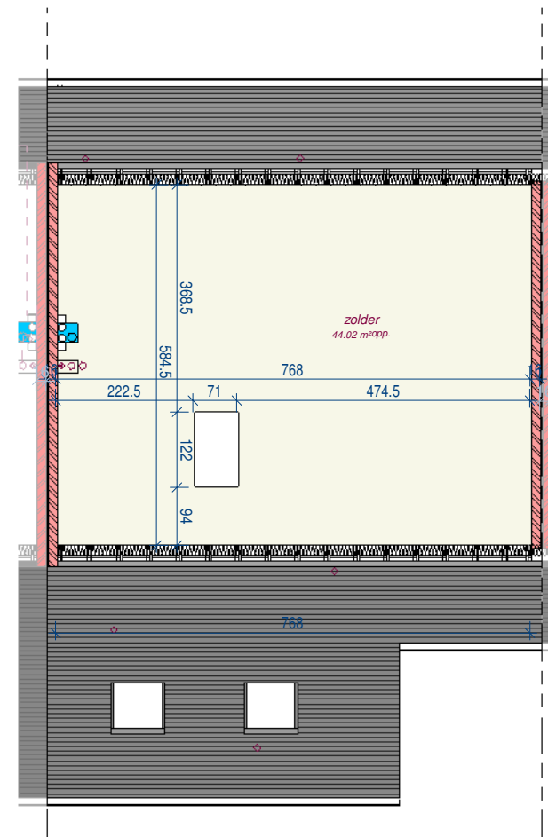
2de verdieping
