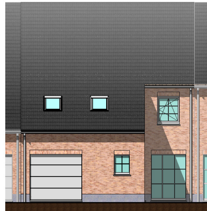
voorgevel
