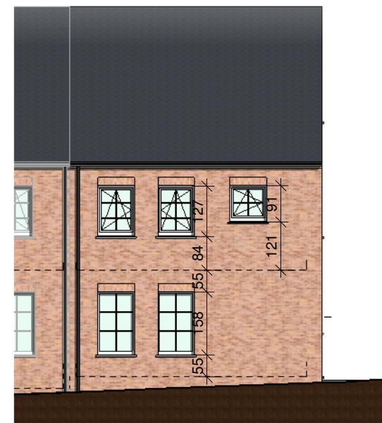
voorgevel
