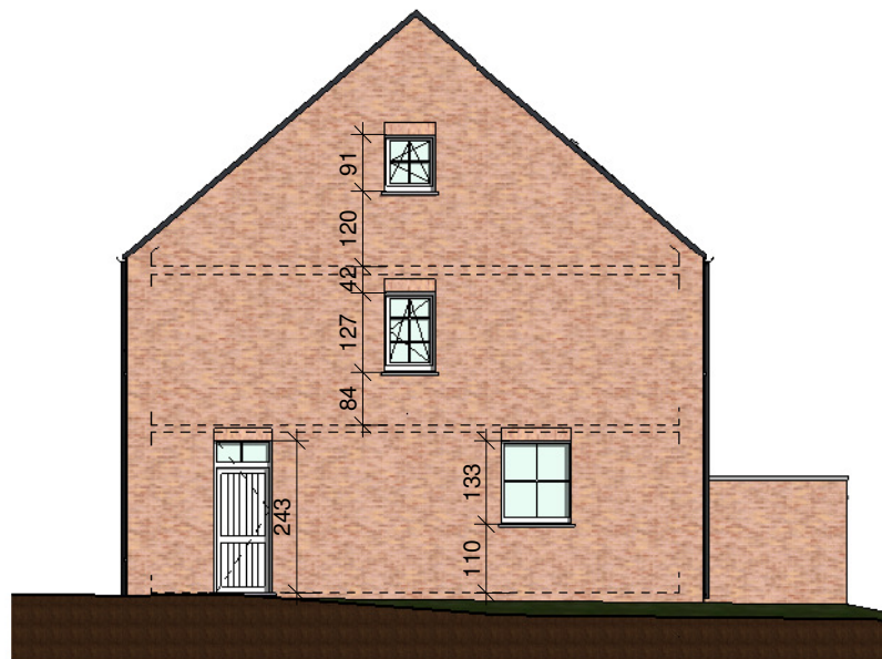
gevel rechts
