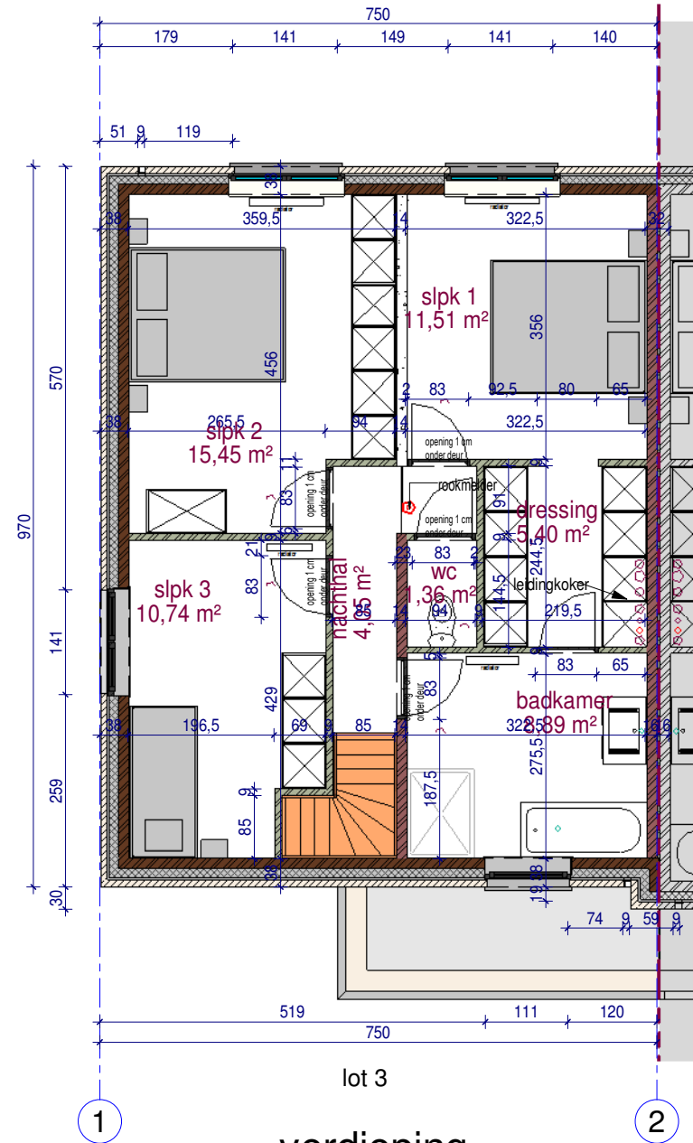
verdieping
