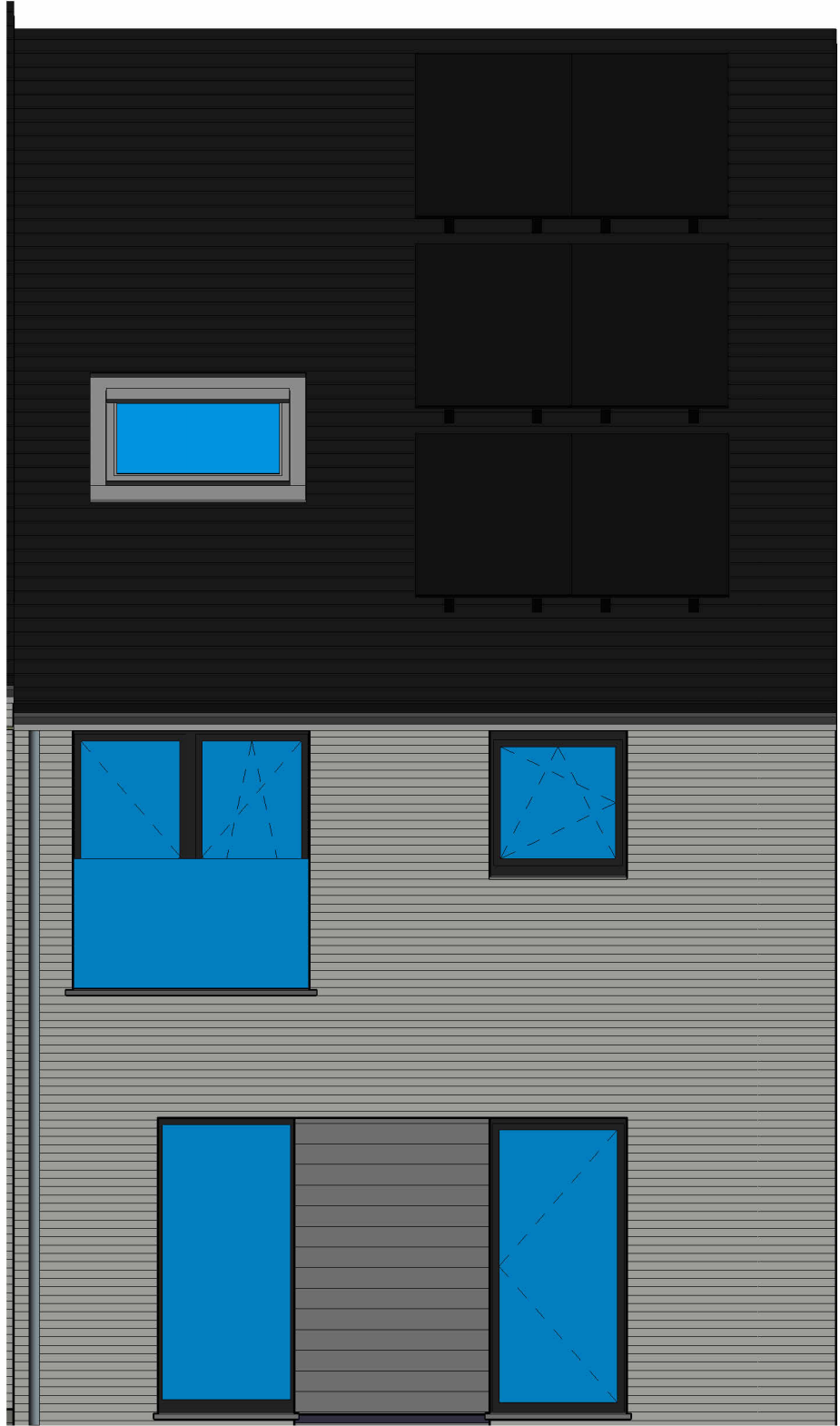
1 Voorgevel lot 47 1 : 50
