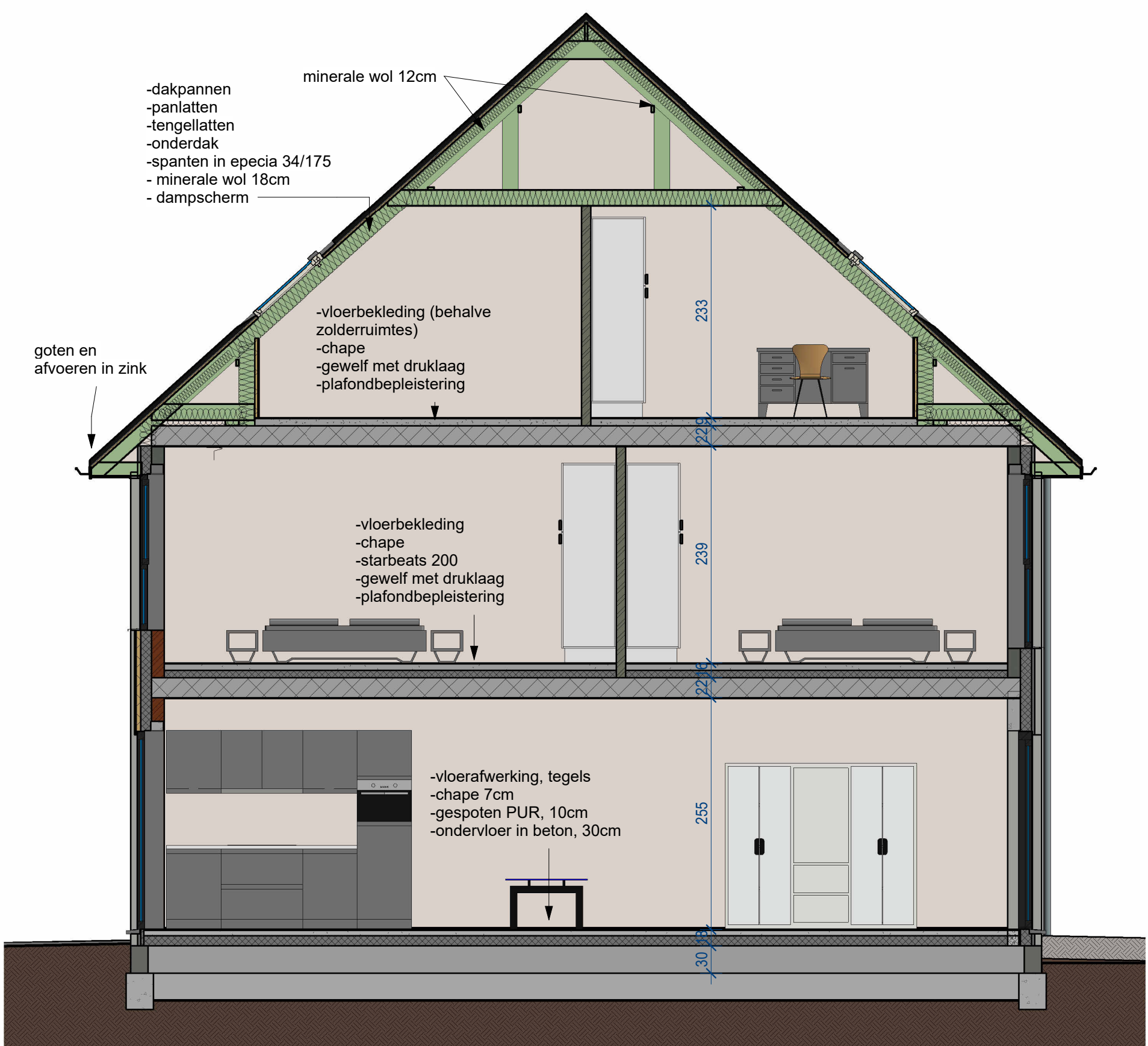
9 Snede VK 47 1 : 50
