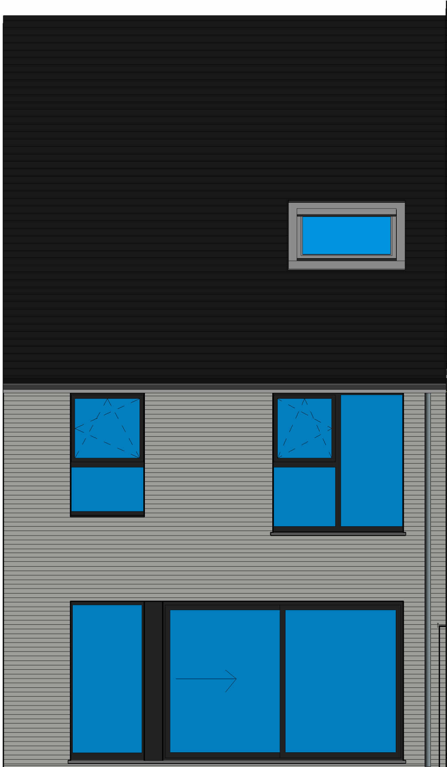
2 Achtergevel lot 47 1 : 50
